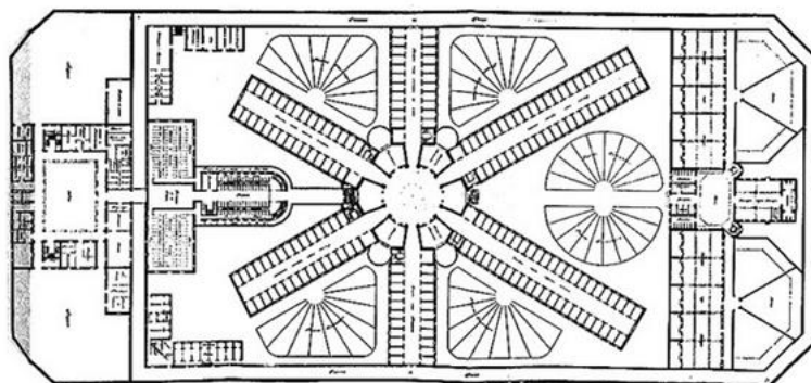
Figura 7. Plano de la Cárcel Modelo de Barcelona.
