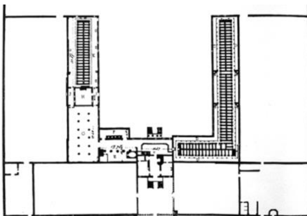
Figura 6. Plano de la Penitenciaría de Auburn.
